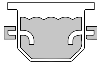
Fossa settica
